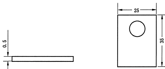
图 2 试验钢板的尺寸及形状
