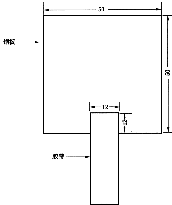
图 1 试件的形状和尺寸
