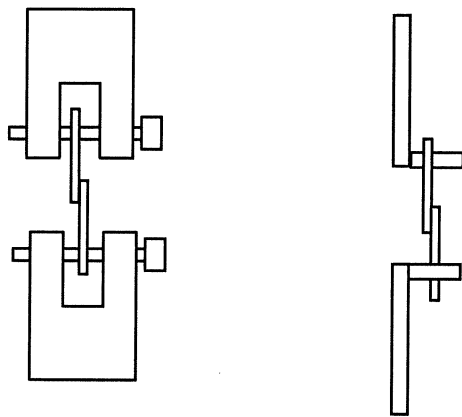
图 3 测试夹具形状示意图
